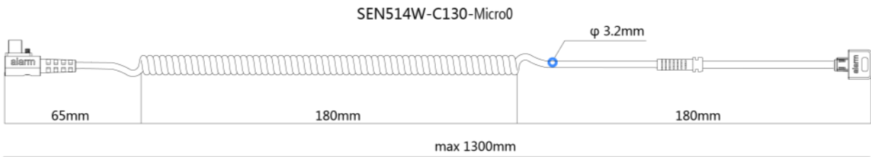
侧弯出线白色弹簧线Micro正 SEN514W-C130-Micro0
