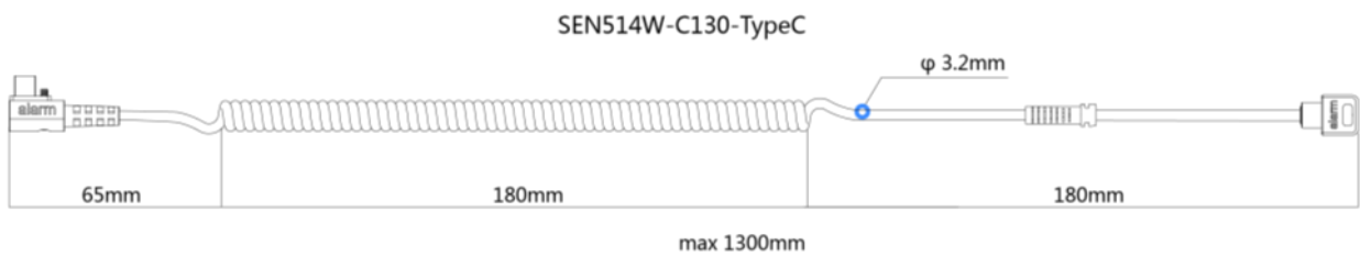
侧弯出线白色弹簧线TypeC头 SEN514W-C130-TypeC
