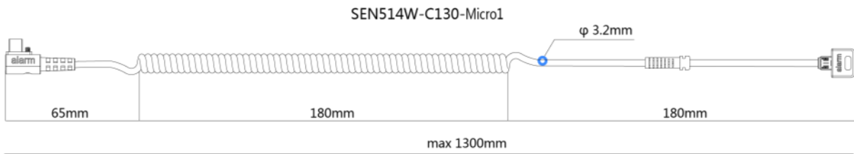
侧弯出线白色弹簧线Micro反 SEN514W-C130-Micro1
